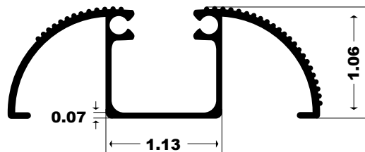
359 - WALKOVER
