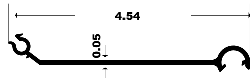
371 - BLADE
