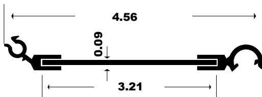
313 - CLEAR BLADE
